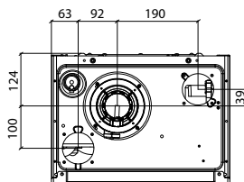
Rozmerová schéma kotla ENBRA FORMENTERA
