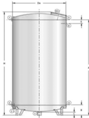
Pro objem nádrže od 3000 do 15 000 litrů.
