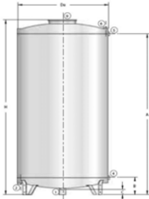
Pro objem nádrže od 125 do 2000 litrů.
